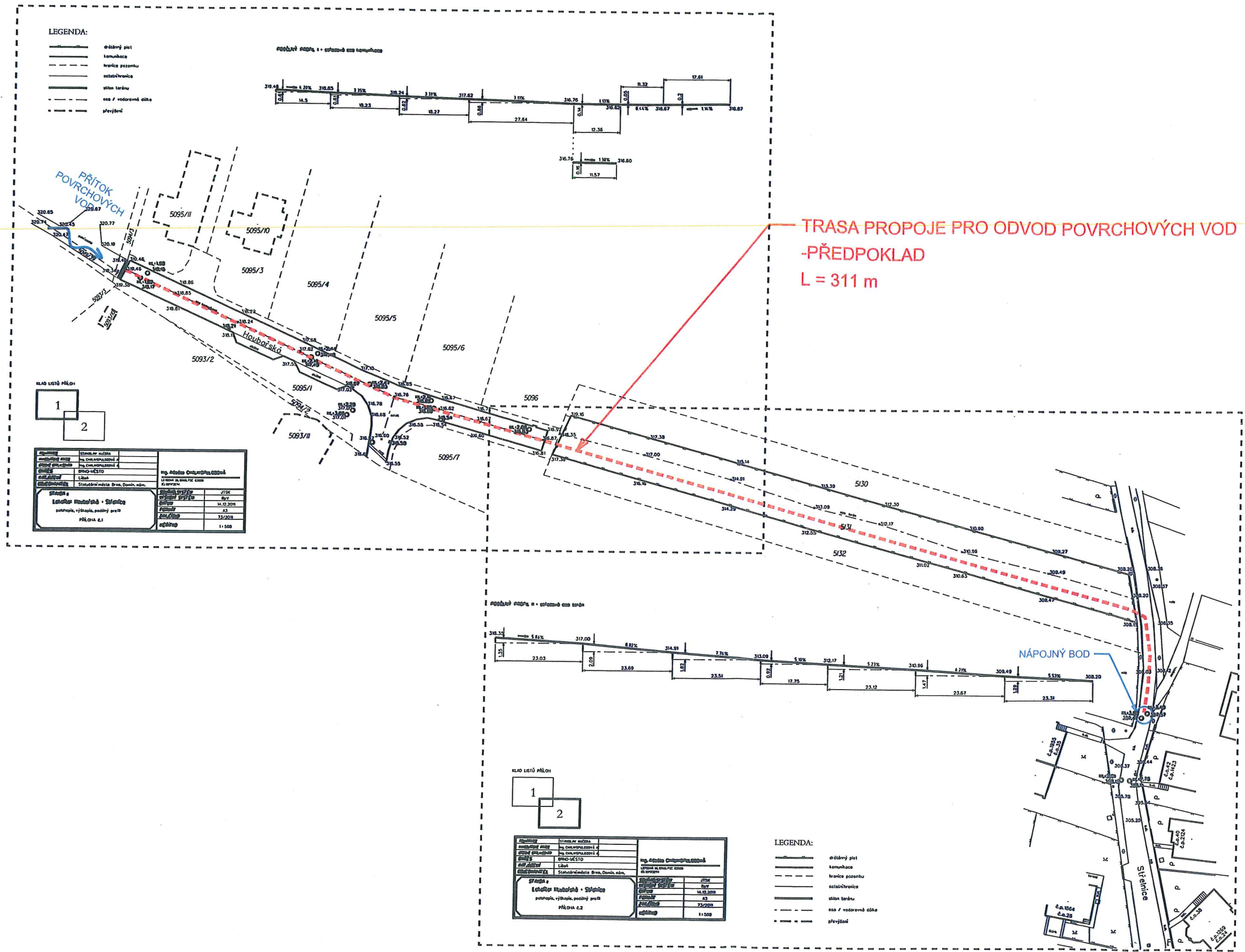
B.3 - SITUACE LOKALITY M 1 : 1 000
