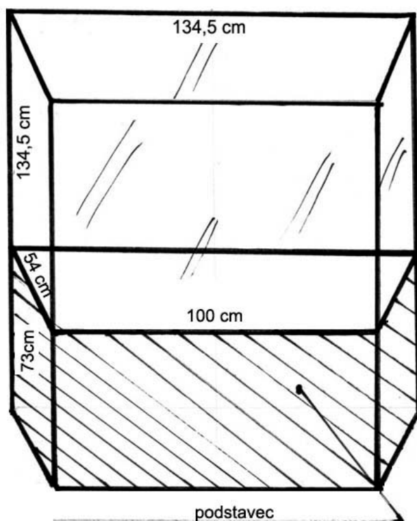
orientační plánec vnitřních rozměrů vitrin
